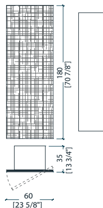
BD 27 M hanging unit - contenitore pensile - hängeschrank - élément mural - Навесной шкаф
