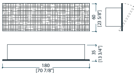
BD 37 M hanging unit - contenitore pensile - hängeschrank - élément mural - Навесной шкаф
