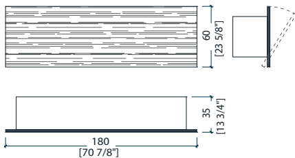
BD 37 R hanging unit - contenitore pensile - hängeschrank - élément mural - Навесной шкаф
