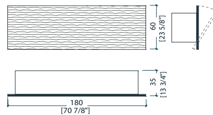
BD 37 O hanging unit - contenitore pensile - hängeschrank - élément mural - Навесной шкаф
