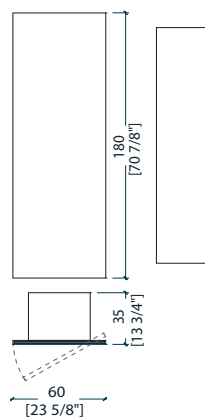
BD 27 RA hanging unit - contenitore pensile - hängeschrank - élément mural - Навесной шкаф
