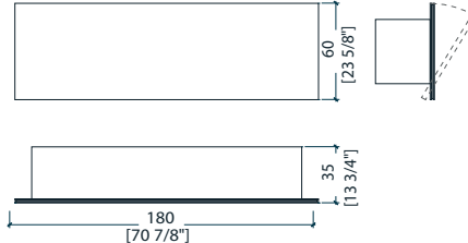
BD 37 RA hanging unit - contenitore pensile - hängeschrank - élément mural - Навесной шкаф
