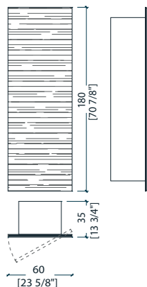
BD 27 R hanging unit - contenitore pensile - hängeschrank - élément mural - Навесной шкаф
