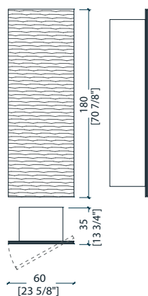
BD 27 O hanging unit - contenitore pensile - hängeschrank - élément mural - Навесной шкаф
